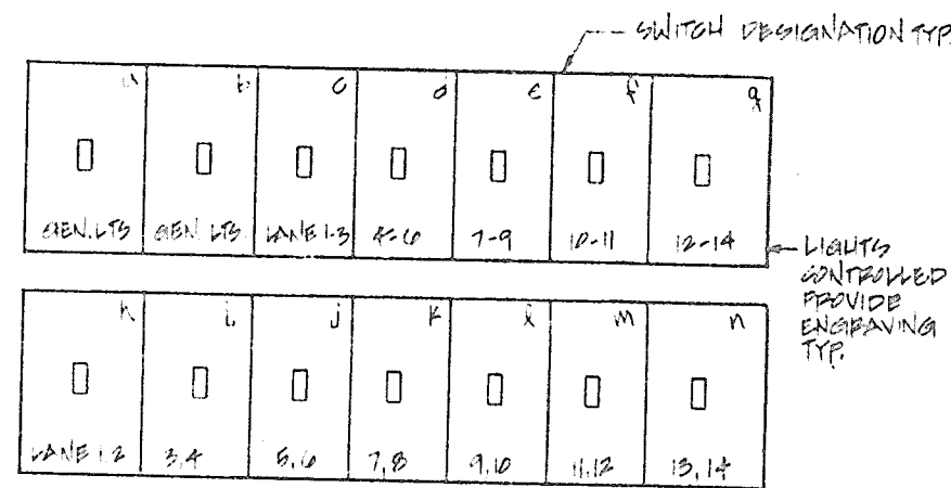
FILING LANE SWITCH BANK ELEVATION N.T.S.
