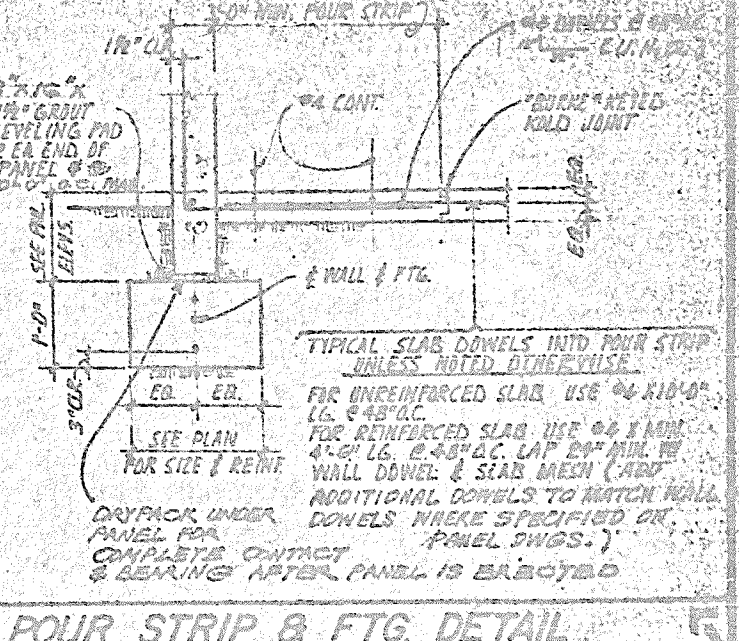
POUR STRIP & FTG. DETAIL
